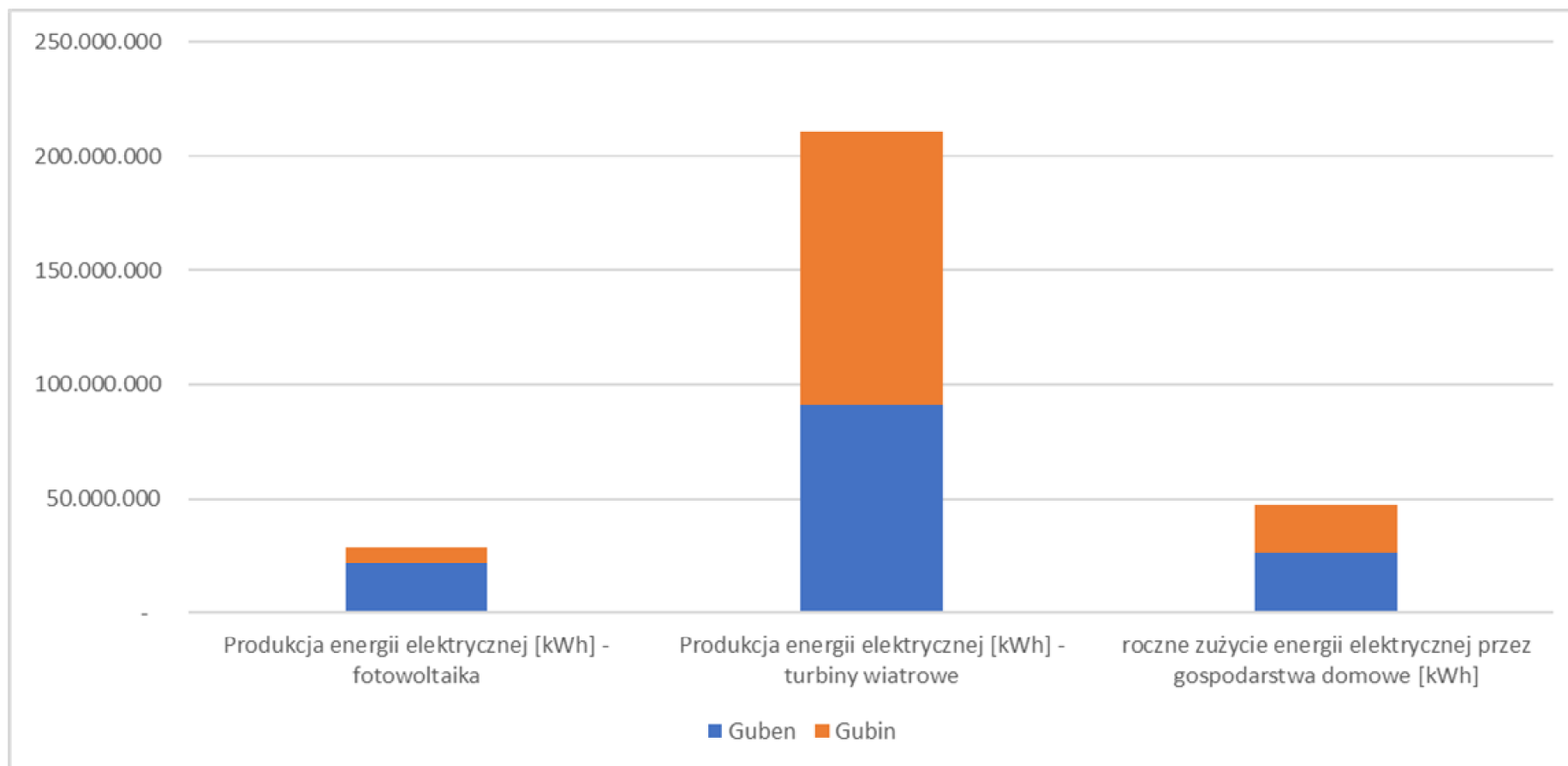
Rysunek 23: Produkcja energii elektrycznej z odnawialnych źródeł energii (fotowoltaika - PVA i turbiny wiatrowe - WKA) w Gubinie i Guben oraz roczne zużycie energii elektrycznej przez gospodarstwa domowe w Gubinie i Guben. Źródła: Bundesnetzagentur MaStR, LfU Brandenburg – LUIS, Windkraftanlagen, DEStatis Private Haushalte und Umwelt, GUS: Zużycie energii w gospodarstwach domowych, StatBB: Zeitschrift für amtliche Statistik Berlin Brandenburg, roczn. 14.
